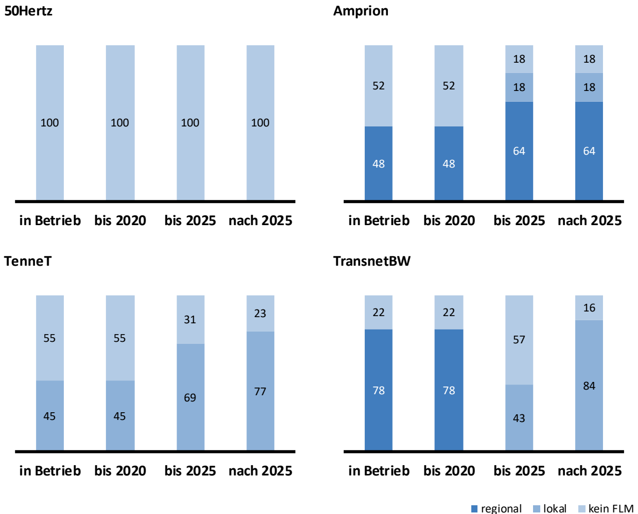
Abbildung 43: Anteil am Freileitungsmonitoring im Höchstspannungsnetz (Angaben für die 220kV-Ebene in Prozent)
